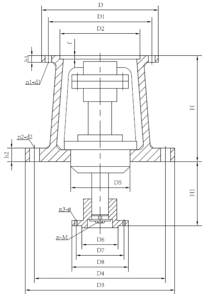
TJA 型 (新标) 机架主要参数及尺寸
