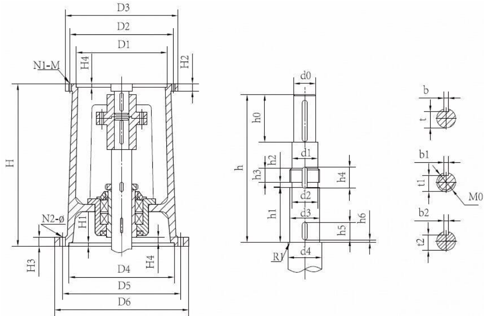
JXD 型单支点机架主要参数及尺寸
