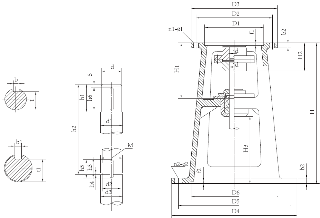
JXLD 型 (74 标) 机架主要参数及尺寸
