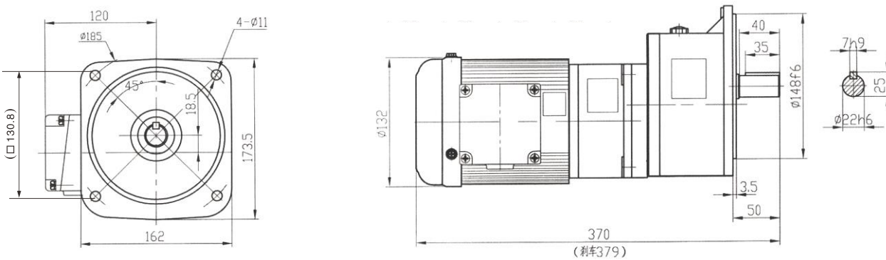
CV28+CV18-100-250~1800
