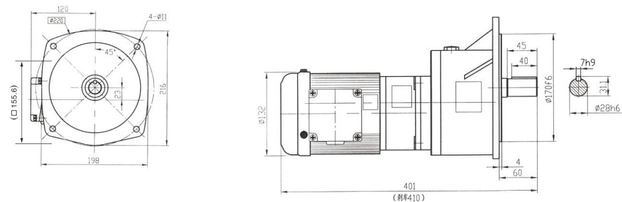
CV28+CV18-100-250~1800
