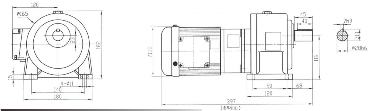
CV22+CV18-100-250~1800 輕負載縮框型 Light load miniature frame
